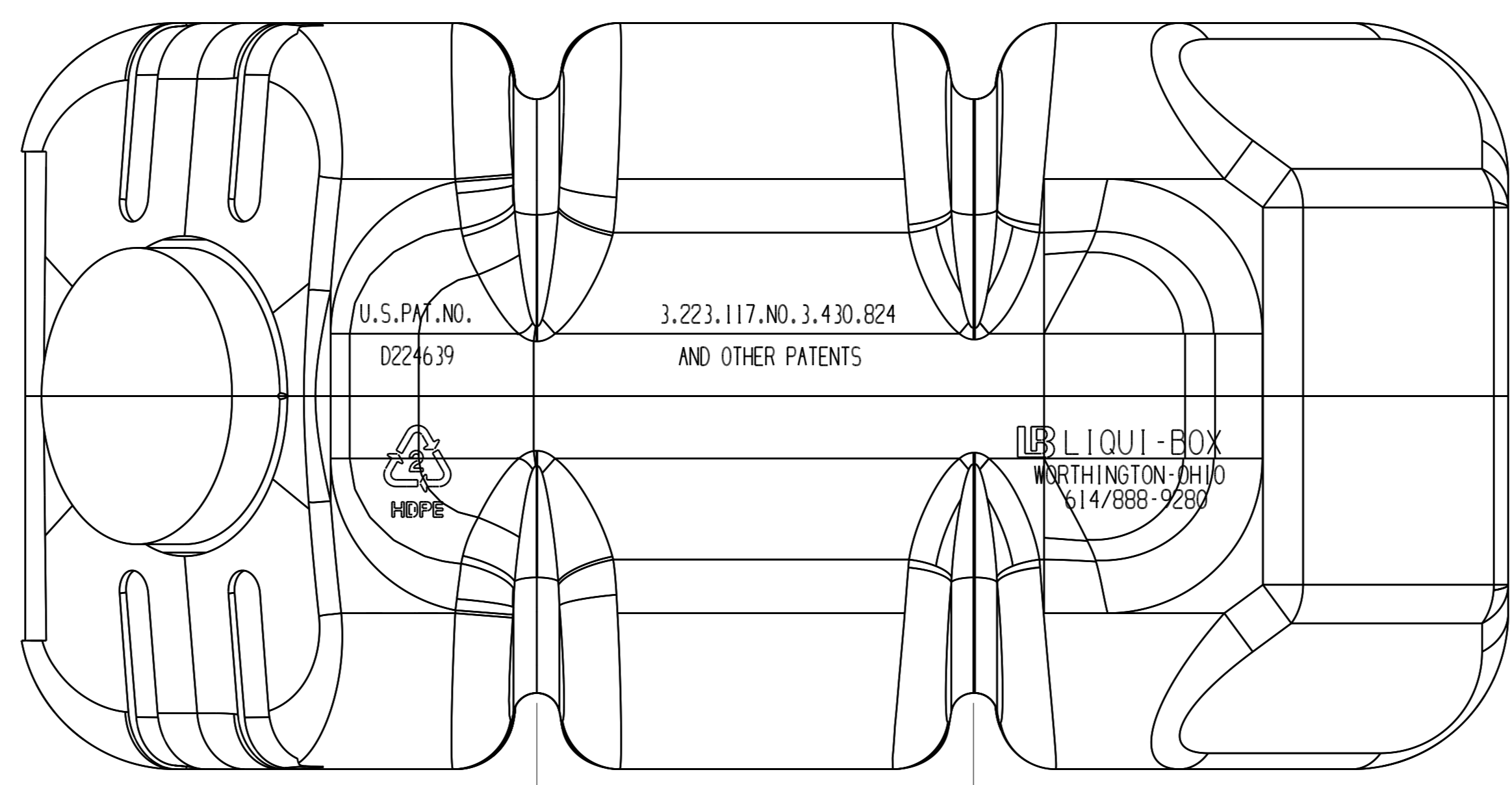
Bottom view Scale: 1:1
