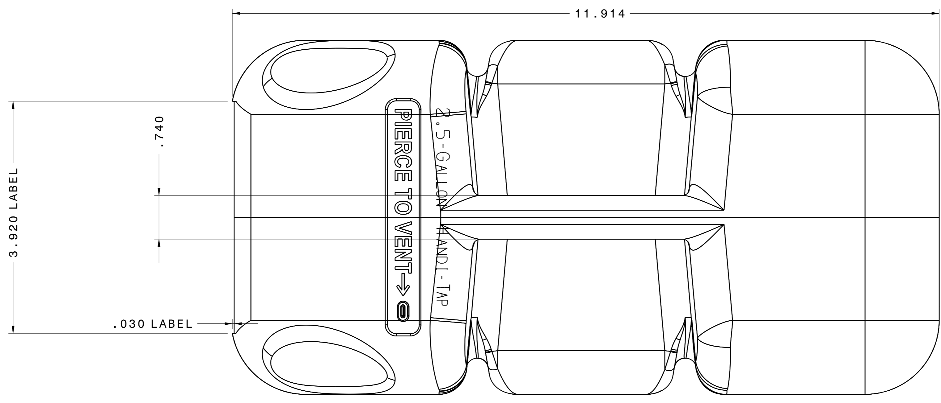
Top view Scale: 1:1
